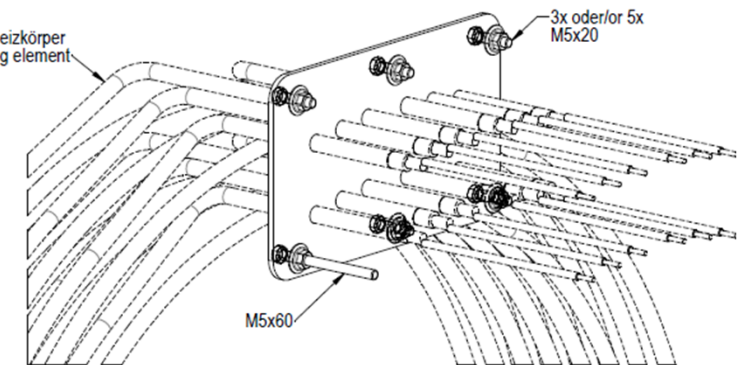
Bolt Material: Stainless steel A2-70 DIN 933
